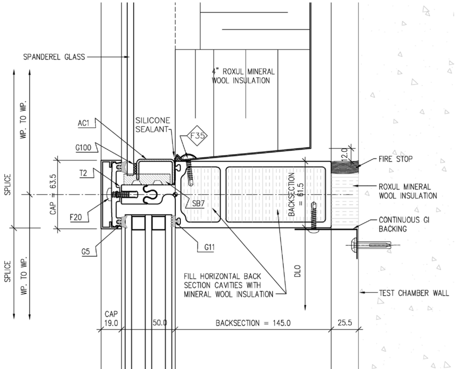
9 2.2 DETAIL SCALE: 1:2
